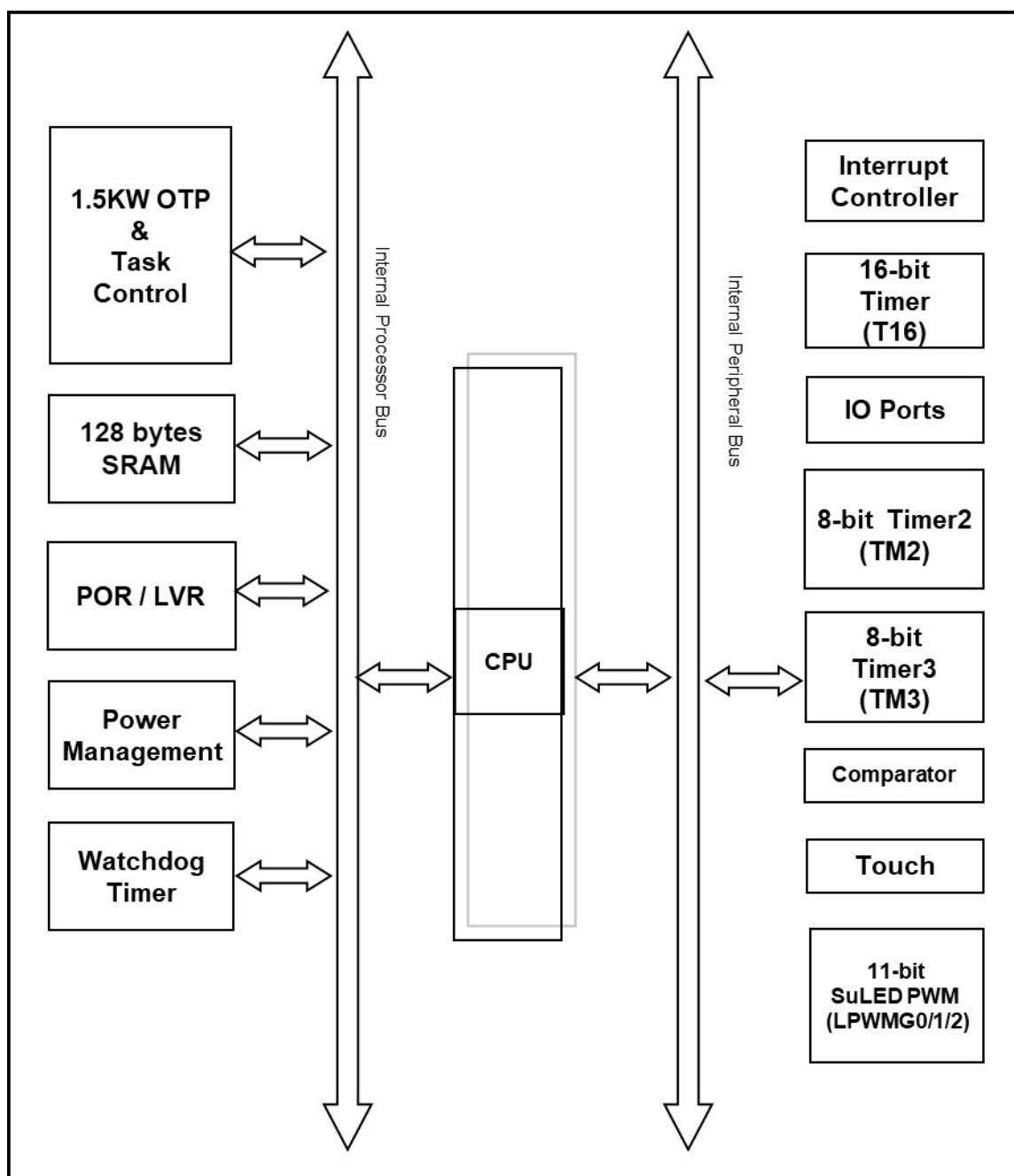
图 1: PMS160B 系统方框图
